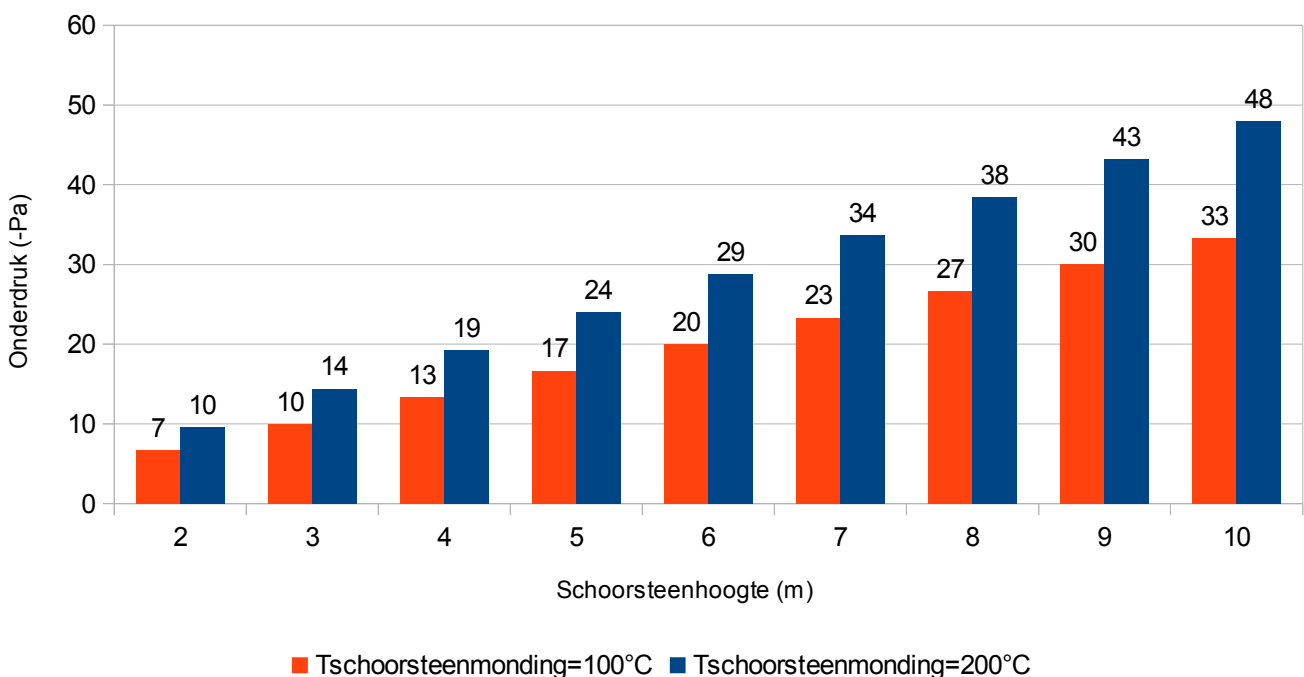
Theoretische onderdruk (trek) bij rechte, warme schoorsteen
